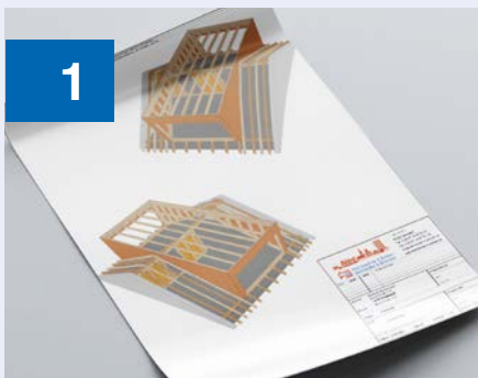
Jedes Bauteil wird präzise konstruiert, sodass die Gaube in einem Stück passgenau montiert werden kann.
